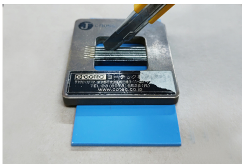
基盤目試験機
